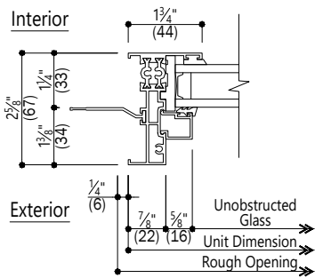
B Jamb 2 Fixed
