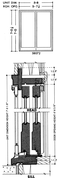
58072 Gliding Door Unit Detail
