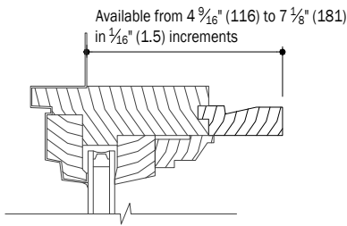
A 4 Extension Jamb
